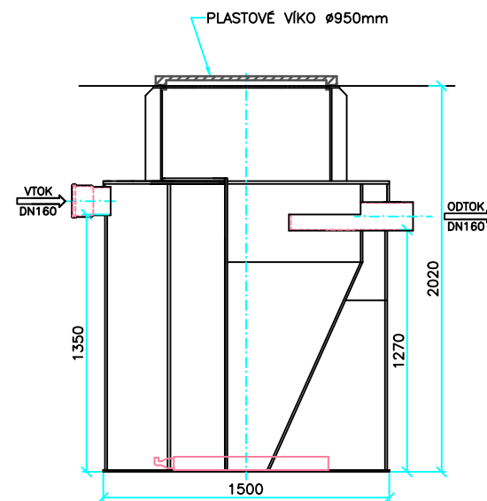
ŘEZ B – B
