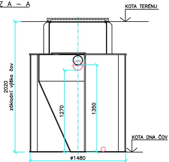
ŘEZ A – A
